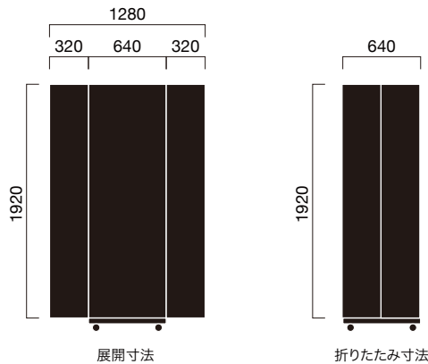
外形寸法
